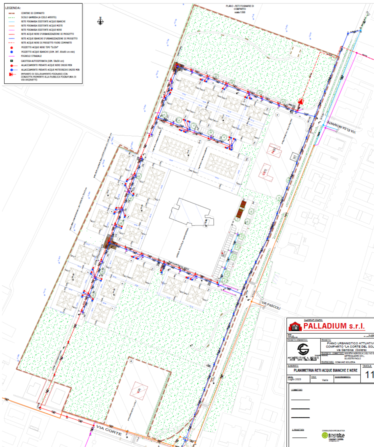
Figura 3 – Lay-out delle reti fognarie a servizio del comparto in esame.
