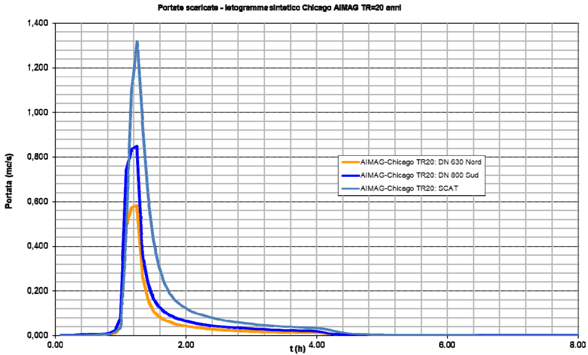
Grafico 1a – Idrogrammi di piena caratteristici in uscita dal comparto – AIMAG Chicago Tr 20 anni
