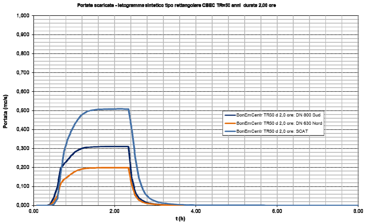
Grafico 1b – Idrogrammi di piena caratteristici in uscita dal comparto – Bonifica Emilia Centrale Tr50 anni durata 2,00 ore
