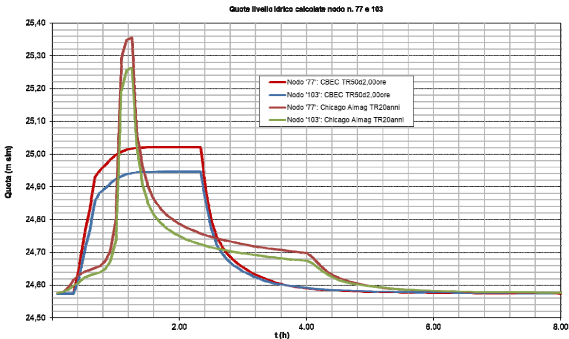
Grafico 2 – Livelli idrometrici interni ai pozzetti (nodo 77 e 103) – quote assolute in m slm.
